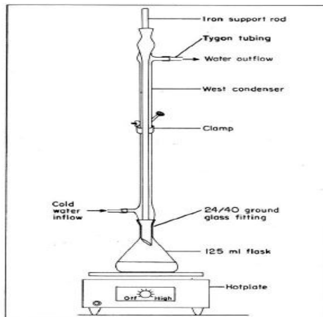
Gambar 1. Peralatan reflux untuk pengukuran COD (sumber: Boyd, 1979)
